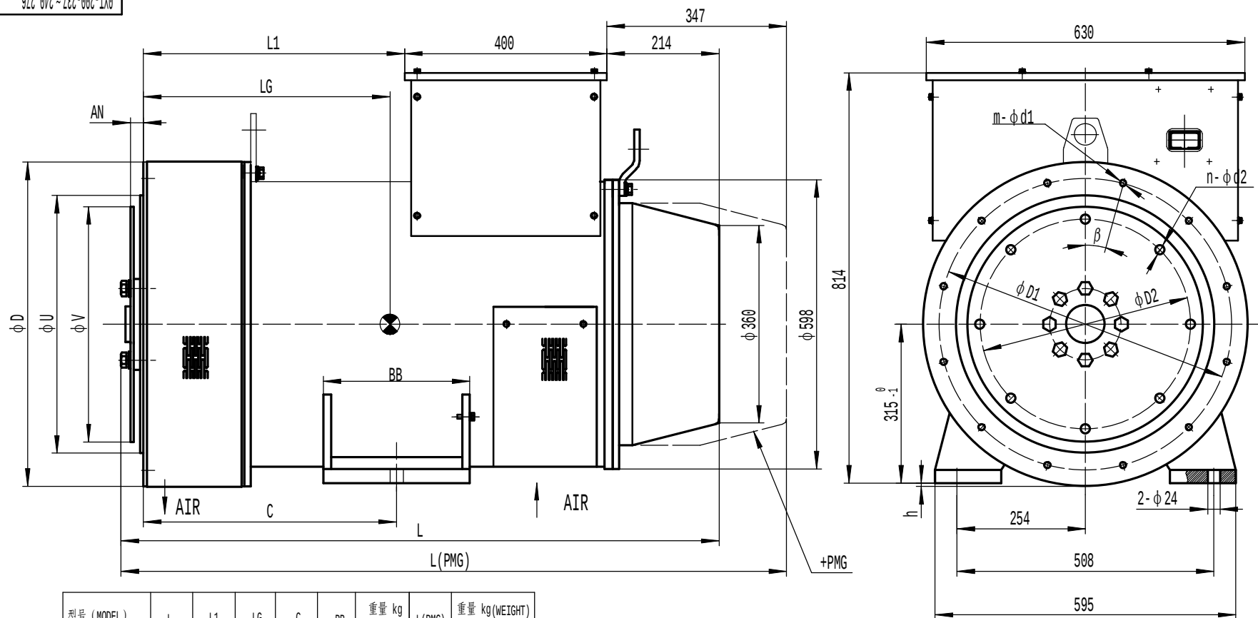
可选连接法兰和驱动盘片SAE号 (FLANGE & COUPLING)
